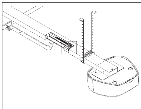
FESTSTELLVORRICHTUNG BEIM ÖFFNEN – ABB. 2A
