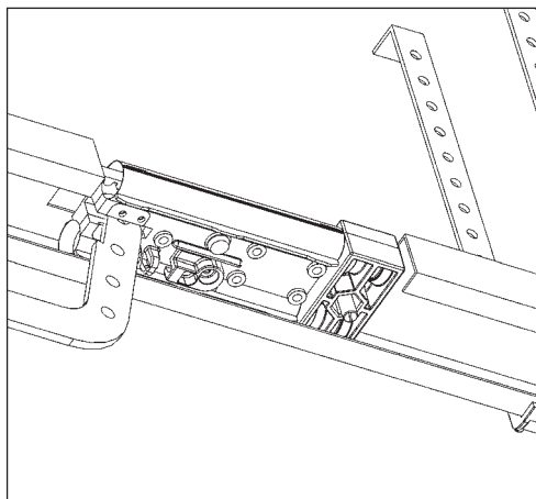
FESTSTELLVORRICHTUNG BEIM ÖFFNEN – ABB. 2A
