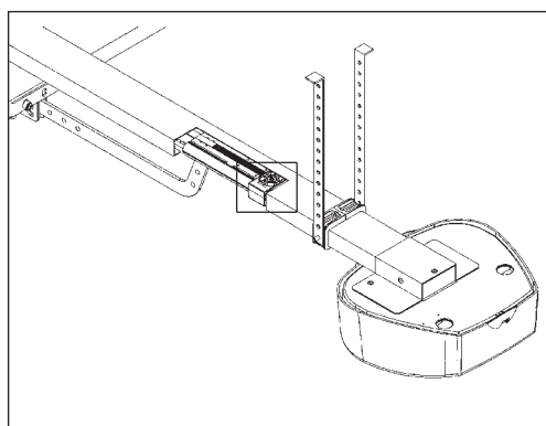
BUTÉE EN OUVERTURE – FIG.2A
