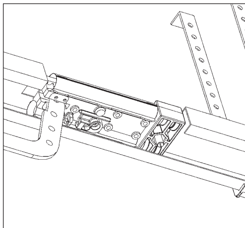
FERMO IN APERTURA - FIG.2 A
