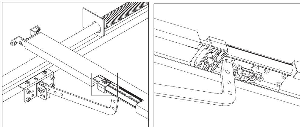
BUTÉE EN FERMETURE – FIG.1A
