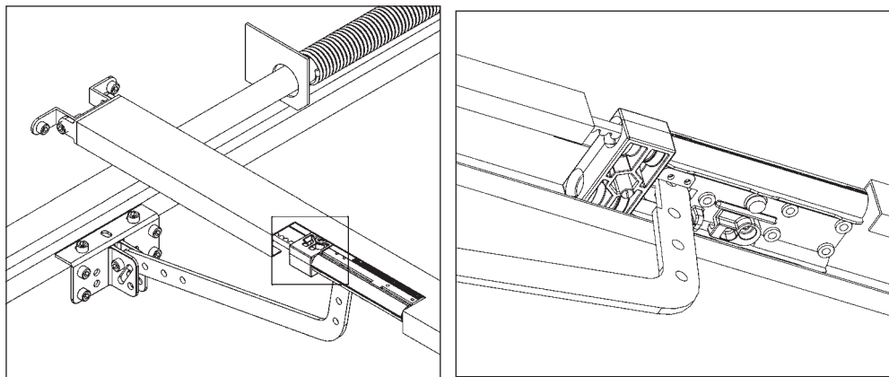
STOP SLUITBEWEGING – AFB.1A
